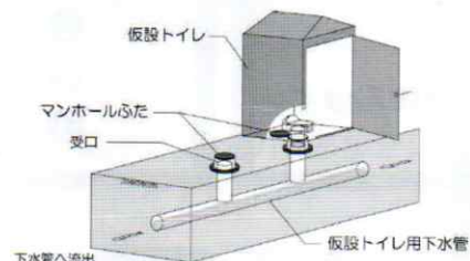
マンホールトイレ構造図 (イメージ)
